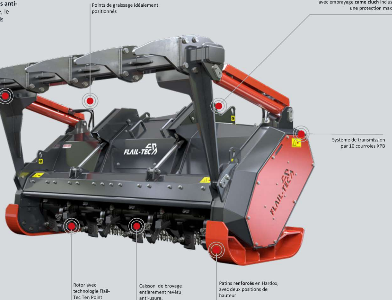
Rabatteur de branches hydraulique avec dents RIPPER en Hardox
